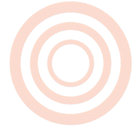
Zen
