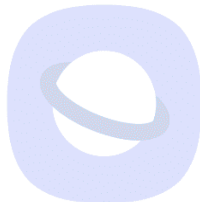
Samsung Internet
