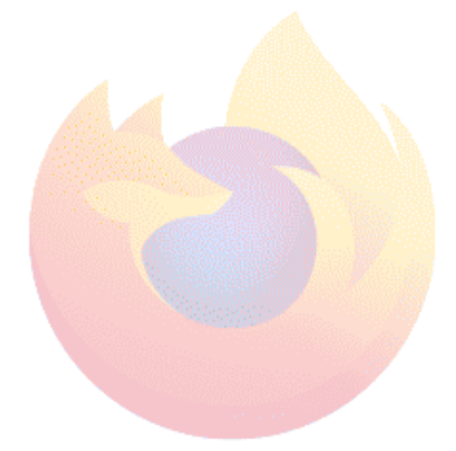
Mozilla Firefox
